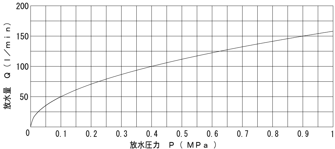
圧力-放水量曲線 流量定数 K=50 ( Q=K\sqrt{10P} )
