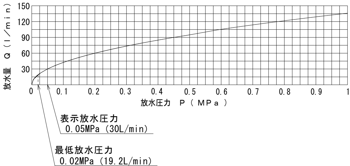
圧力-放水量曲線 流量定数 K=43 ( Q=K\sqrt{10P} )
