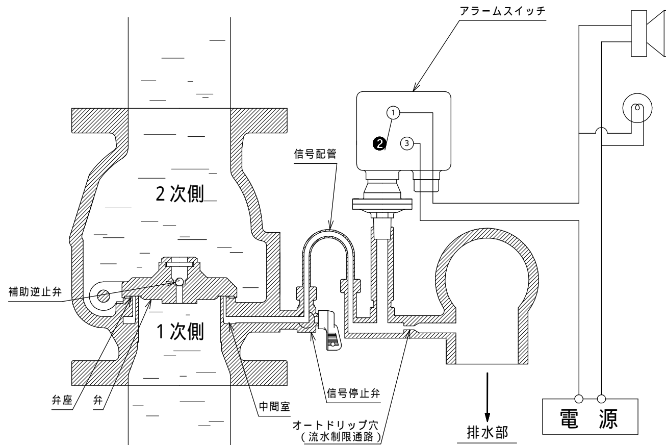
流水検知装置通常状態図
