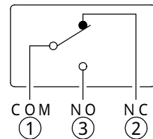
スイッチ内部結線図
