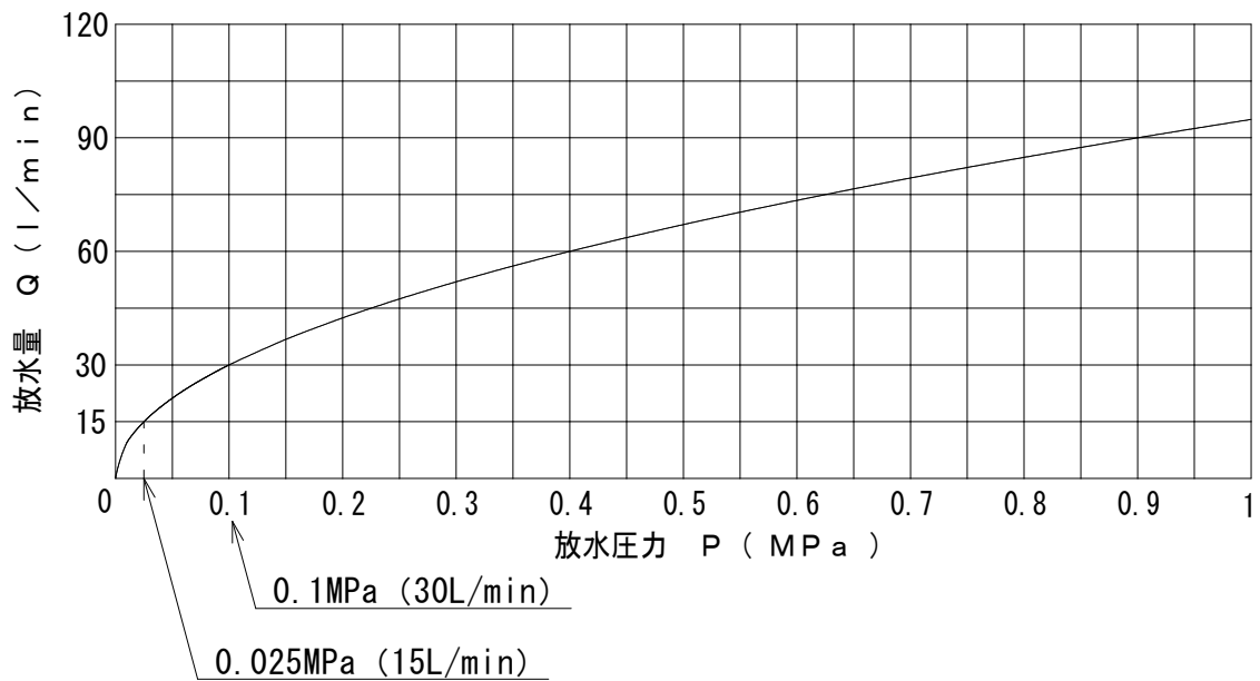
圧力-放水量曲線 流量定数 K=30 ( Q=K\sqrt{10P} )
